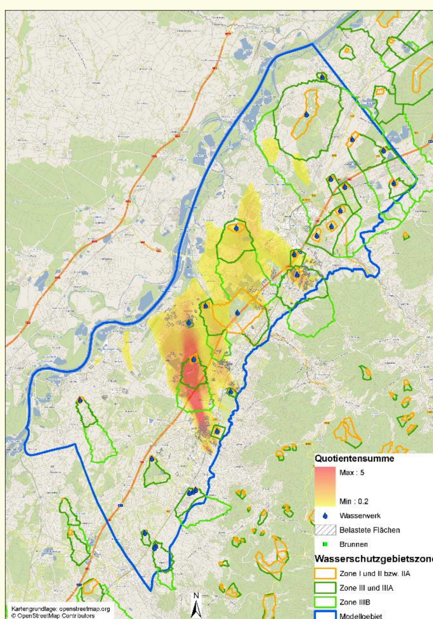
Berechnete PFC-Belastung im oberen Grundwasserleiter Ende 2026. Dargestellt ist die Quotientensumme aus den Konzentrationsverteilungen der Einzelspezies
