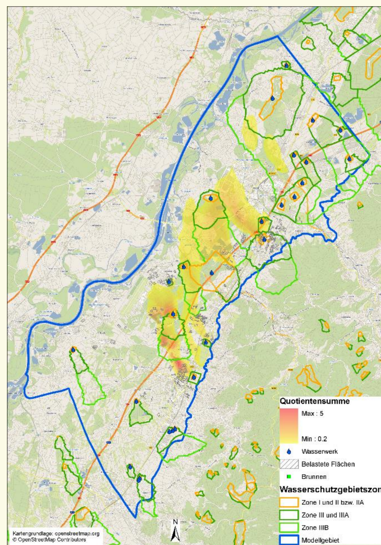
Mit Hilfe des Modells berechnete Quotientensumme im unteren Grundwasserleiter für Ende 2026
